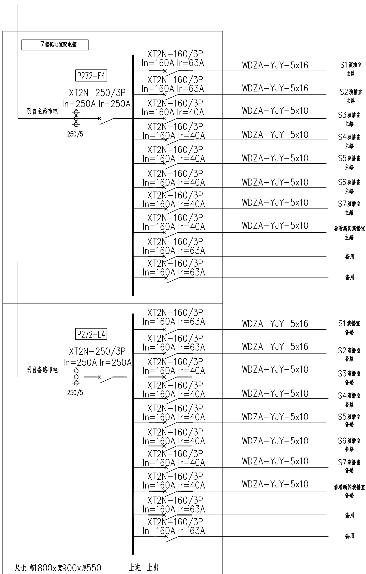
7楼配电室配电箱系统图
