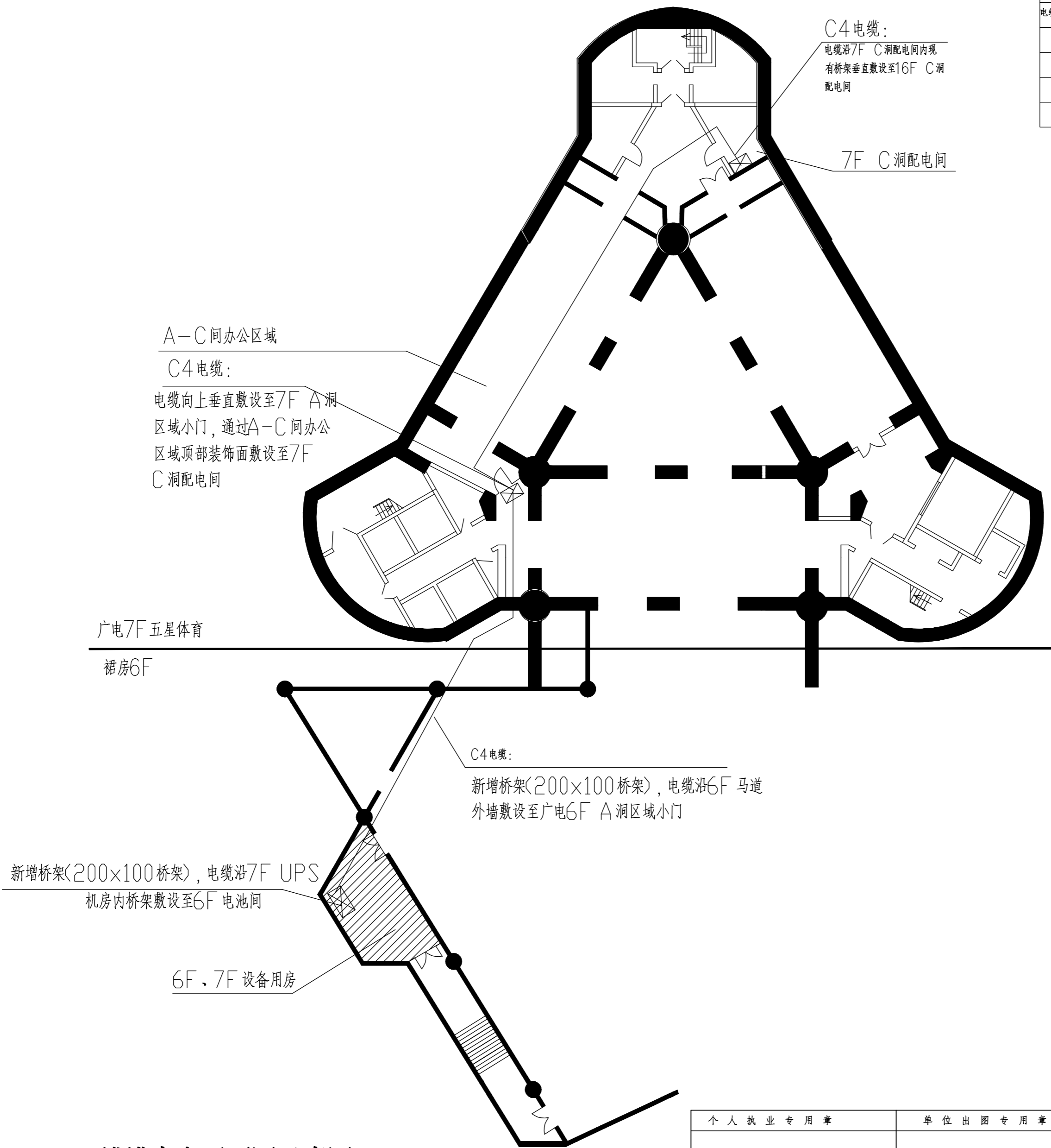
线缆走向平面图示意图二 1:200
